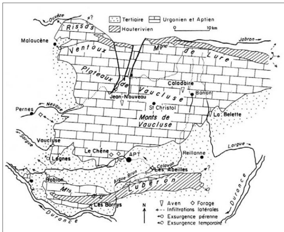
Schéma structural des massifs calcaires à faciès urgonien (Source : Guide géologique régional de Provence)
